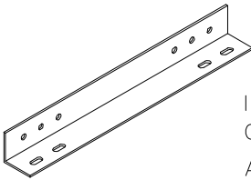
ITEM # 2 QTY: 4 Angle, Incline, 25.5” Long
